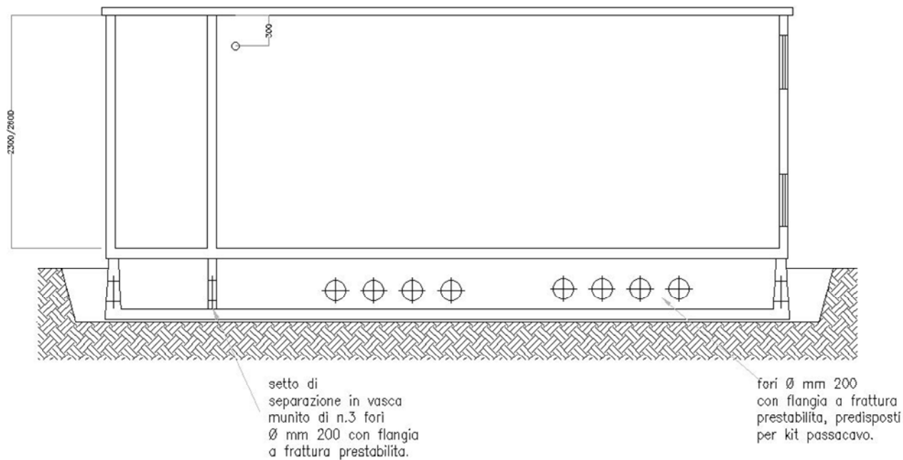
SEZIONE LONGITUDINALE
