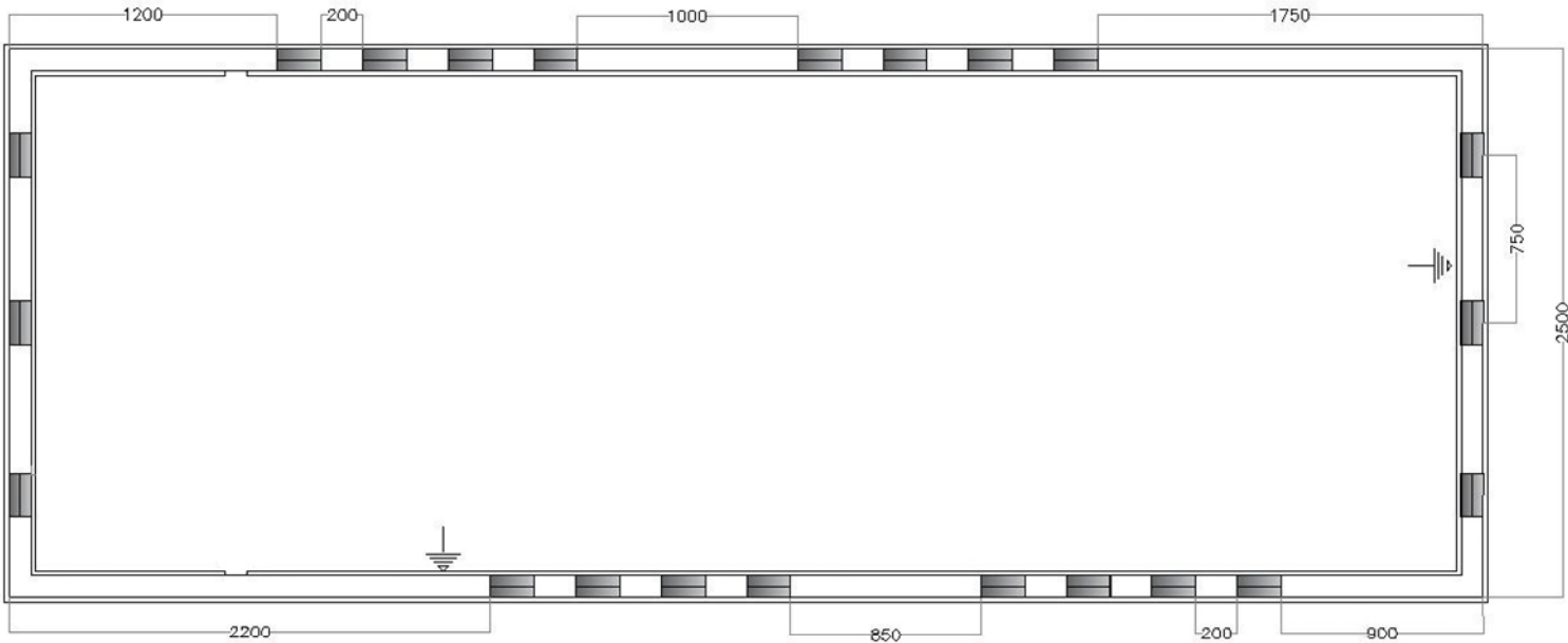
PIANTA BASAMENTO
