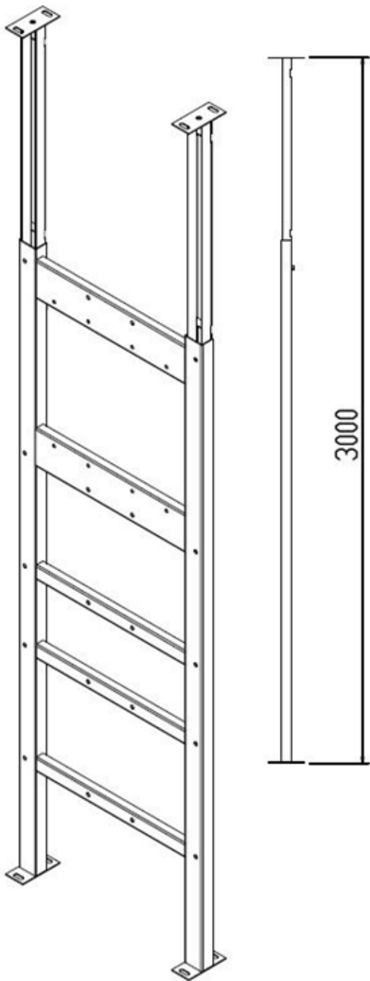
MASSIMA ESTENSIONE
